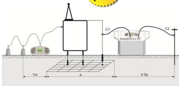
Tension de contact
