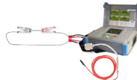
MESURE D'EQUIPOTENTIALITE A COURANT FORT Résolution de 0,1μΩ avec compensation de la température
