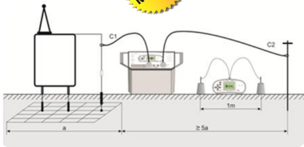
Tension de pas
