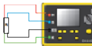
MESURE D'EQUIPOTENTIALITE COURANT FAIBLE
