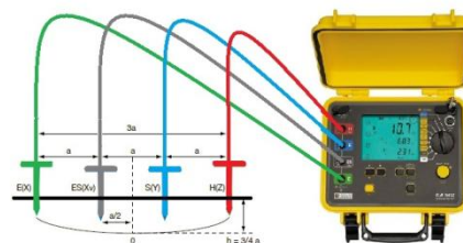
MESURE DE RESISTIVITE DU SOL
