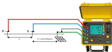
MESURE DE TERRE METHODE 4P
