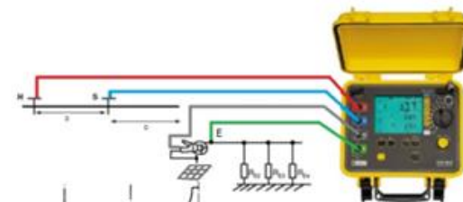
MESURE DE TERRE METHODE 4P SELECTIVE
